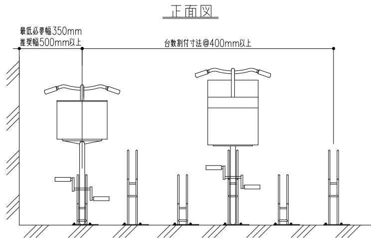
平面式サイクルラック (前輪タイプ) P-1 仕様
